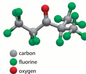
Novec™ 1230 molecule
