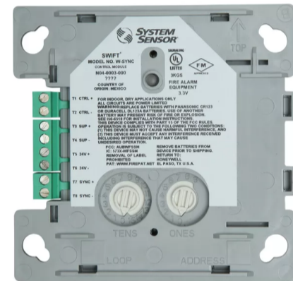
SWIFT® W-SYNC Synchronization Module
